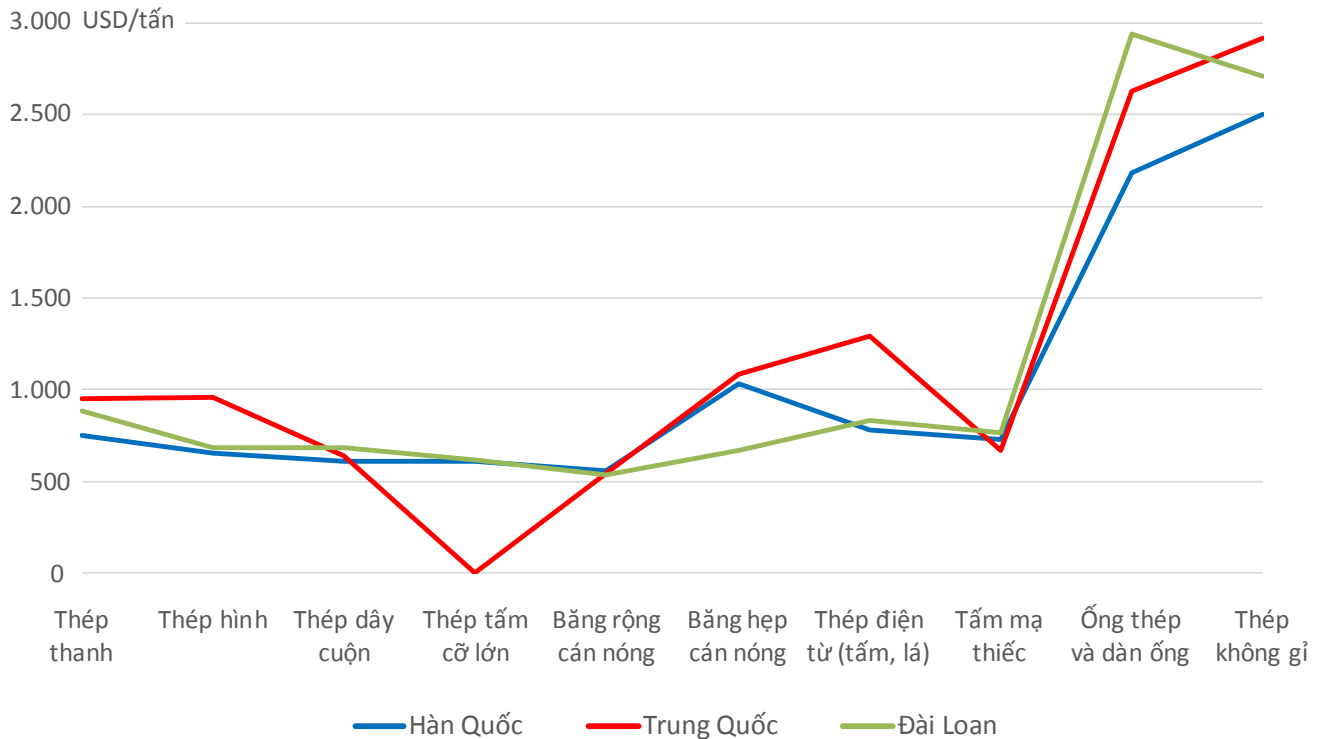
Biểu đồ 14: Giá thép nhập khẩu trung bình tháng 3 của Nhật Bản (Nguồn: Hiệp hội Sắt thép Nhật Bản).
