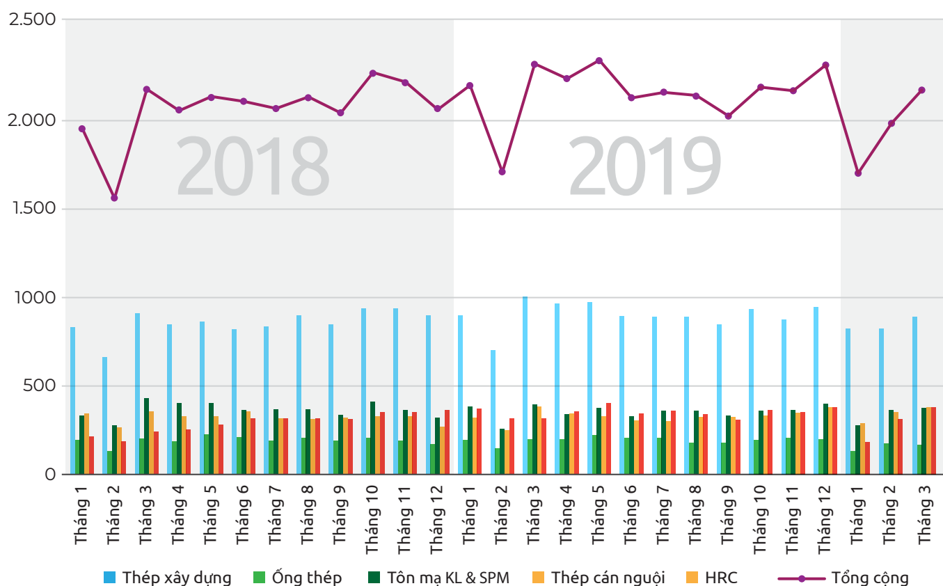
Biểu đồ 22: Tình hình sản xuất thép thành phẩm năm 2020 (Nguồn: Hiệp hội Thép Việt Nam).
