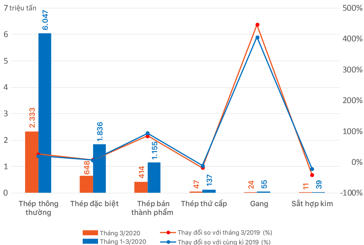
Biểu đồ 4: Các dòng sắt, thép xuất khẩu chủ yếu của Nhật Bản (Nguồn: Nguyễn Thương tổng hợp, Hiệp hội sắt thép Nhật Bản).
