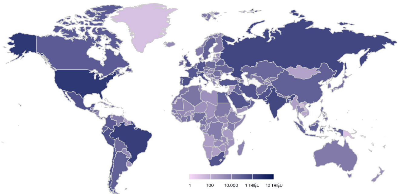
Biểu đồ 3: Diễn biến số ca nhiễm COVID-19 trên toàn cầu (Nguồn: Worldometer).
